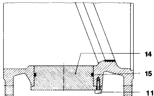
mit Verschlussdeckel / with blind cover
