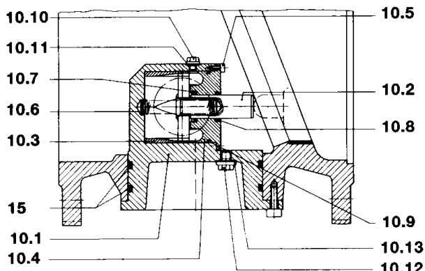
mit innenliegender Endlagendämpfung with internal damper
