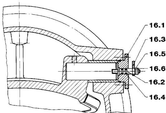
mit Klappenstellungsanzeige/ with position indicator
